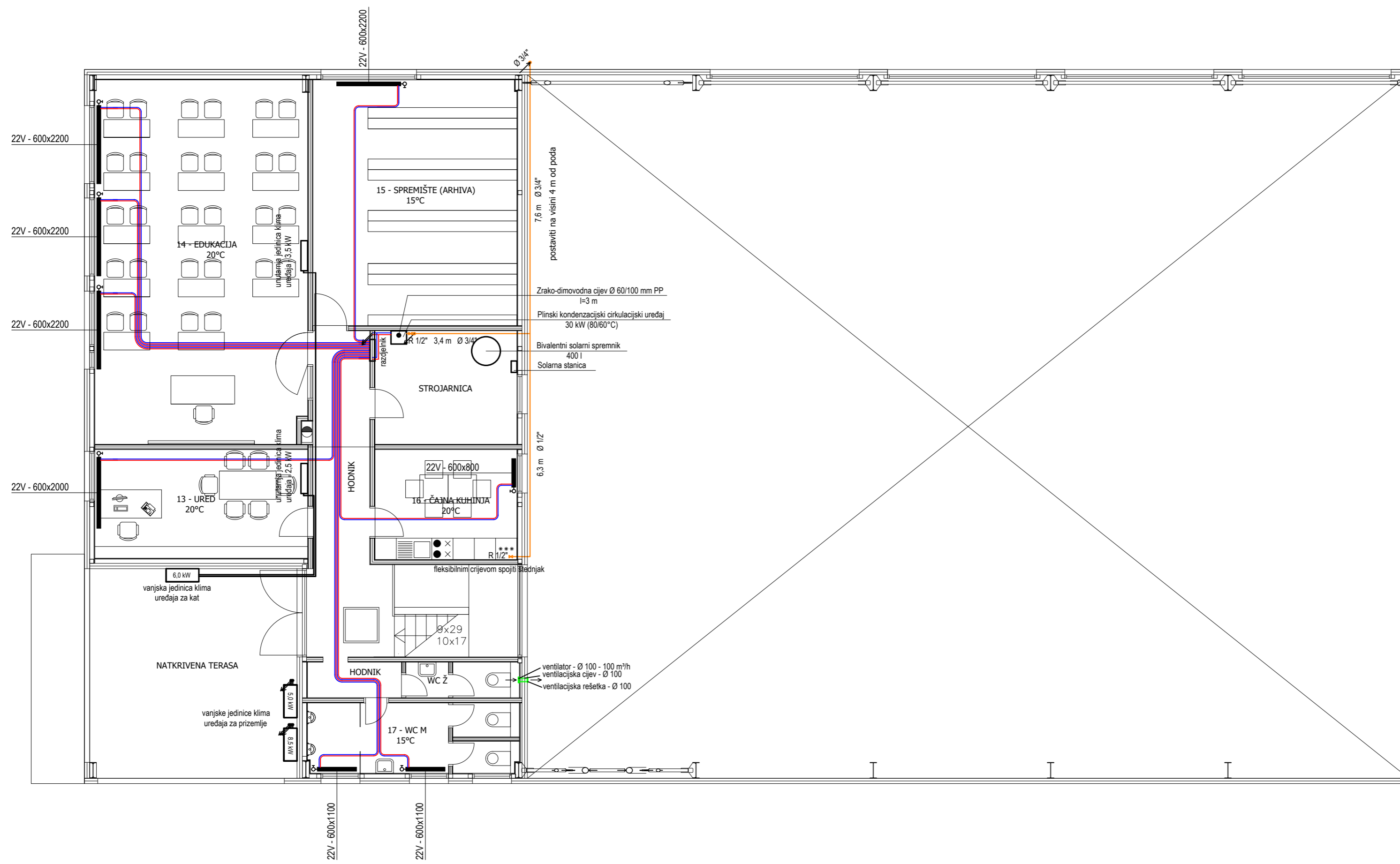
DETALJ - odvod dimnih plinova i dovod zraka
