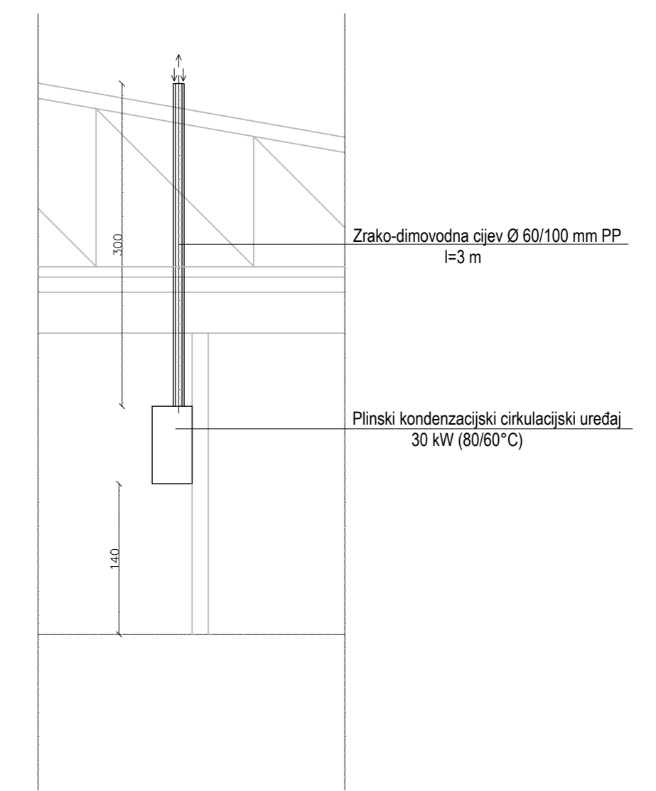
DETALJ - odvod dimnih plinova i dovod zraka
